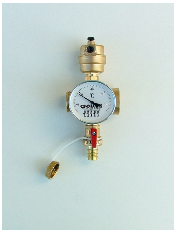
KE 501 tip. komplett végelem 1"-1/2"-1/2"-1/2"
